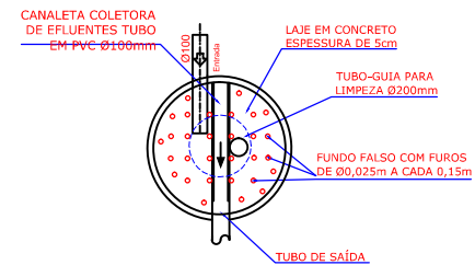
PLANTA BAIXA 02
