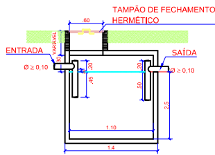
CORTE AA
