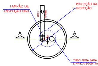
PLANTA BAIXA 01
