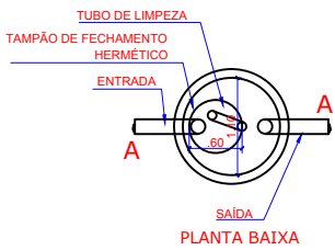
PLANTA BAIXA
