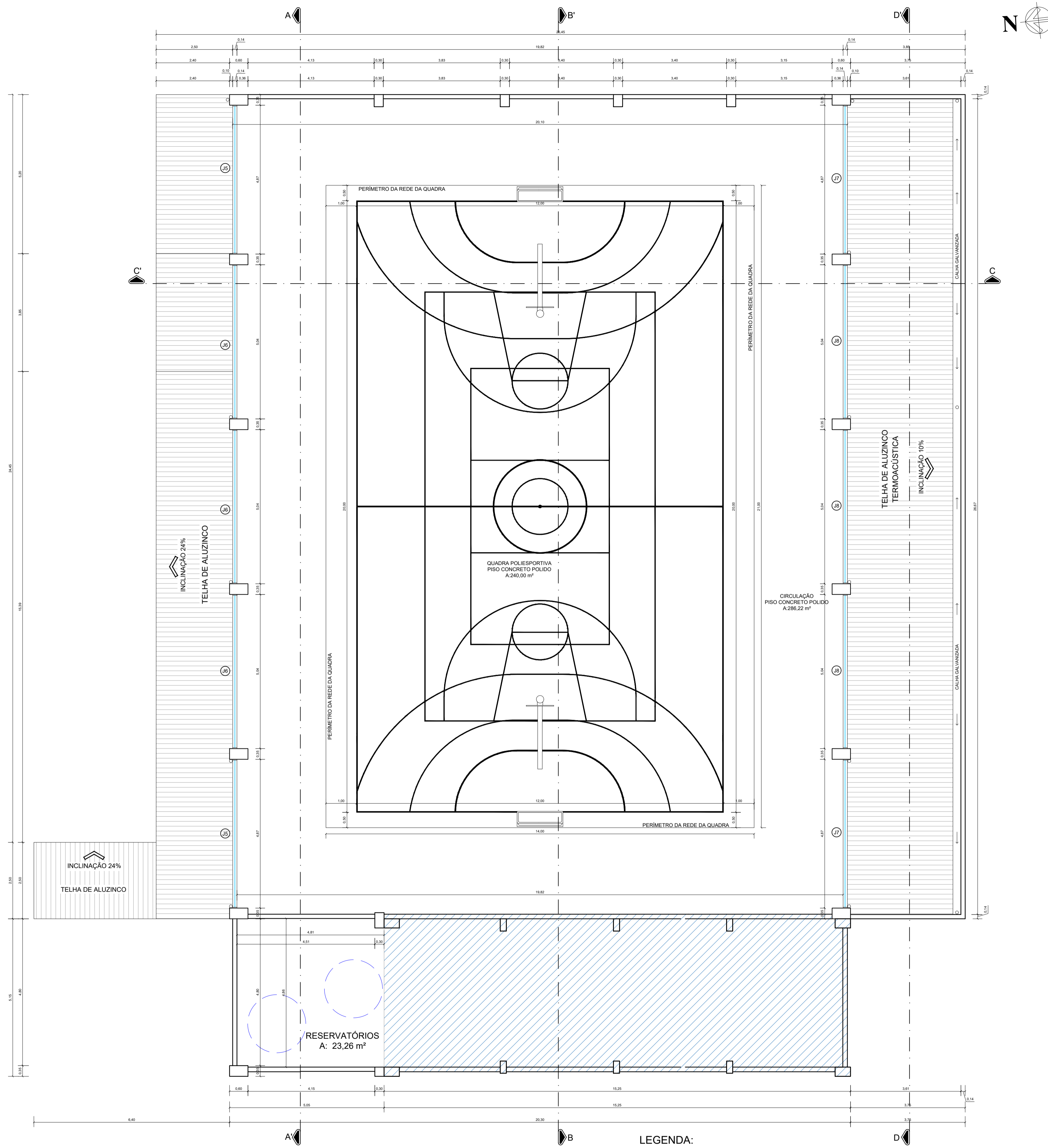
6 PLANTA BAIXA TÉCNICA - RESERVATÓRIOS ESCALA: 1/75
