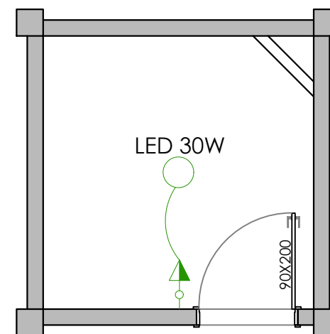
PONTOS ELÉTRICOS ESCALA: 1/50
