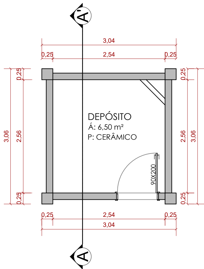
PLANTA BAIXA NÍVEL 0 ESCALA: 1/50
