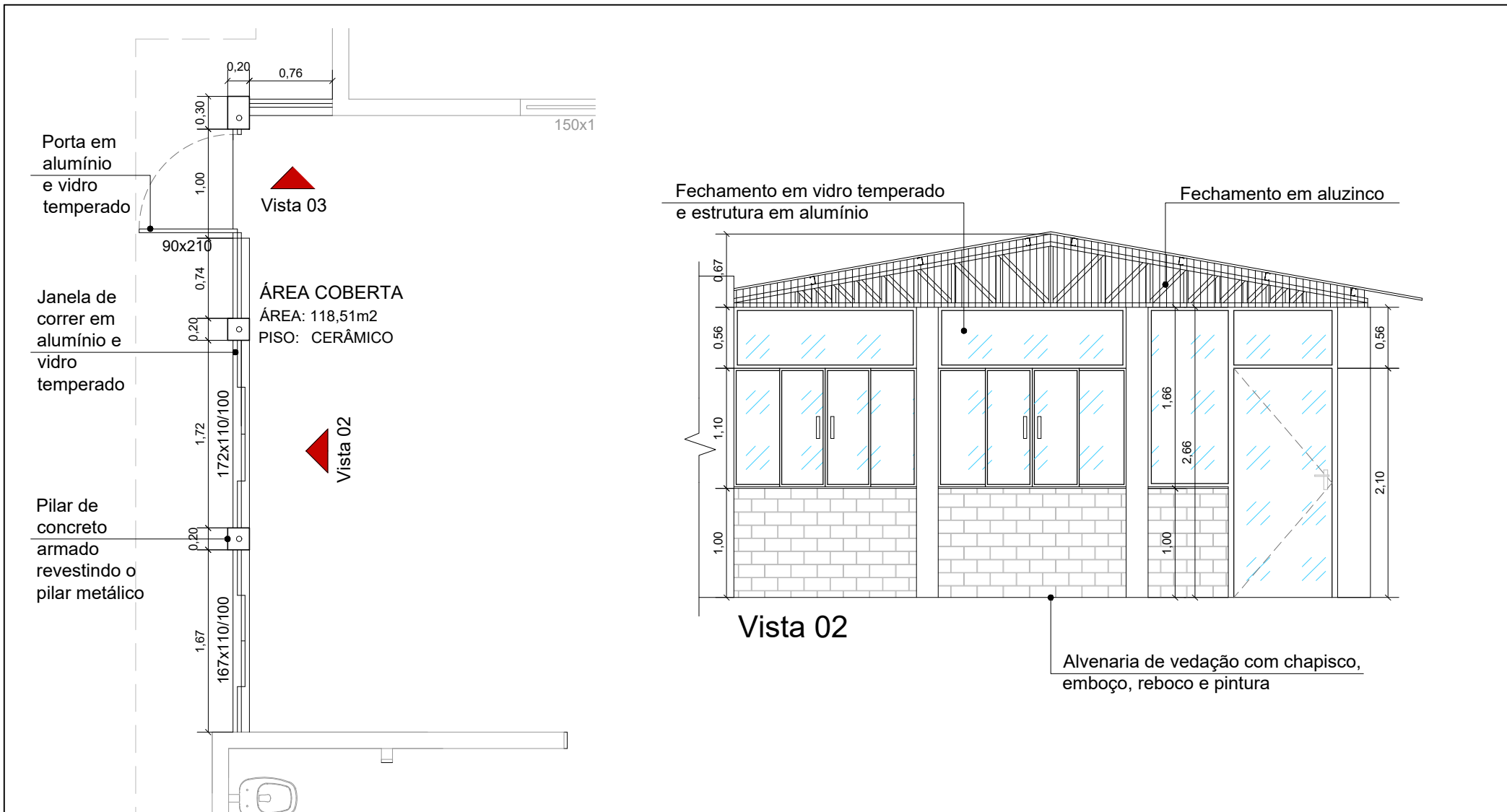
Planta baixa - Fechamento área coberta Escala: 1/50
