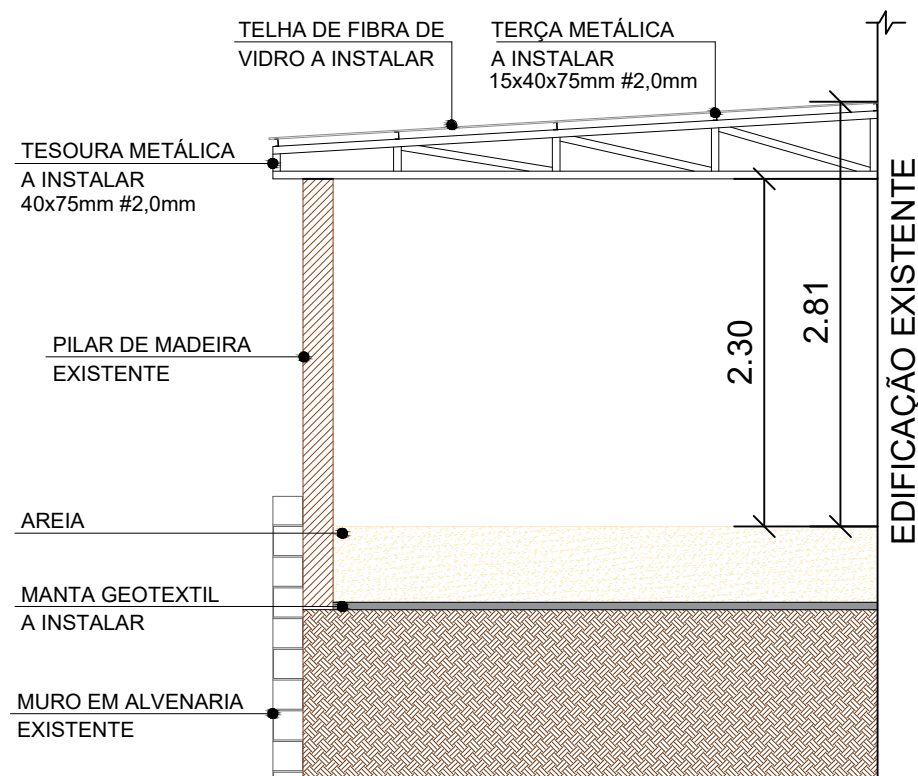
5 CORTE AA' ESCALA: 1/50
