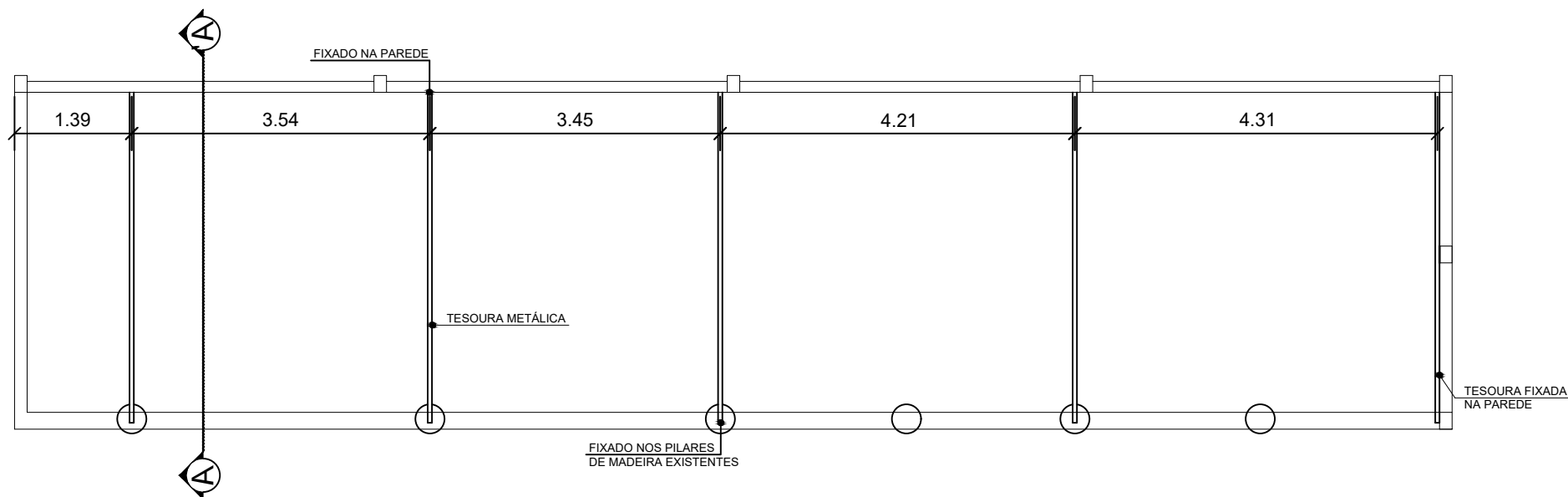
3 PLANTA COBERTURA - TESOURAS ESCALA: 1/75
