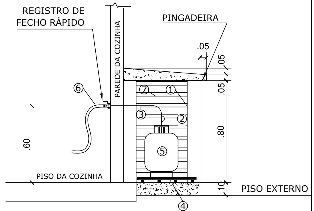
CORTE AA'
