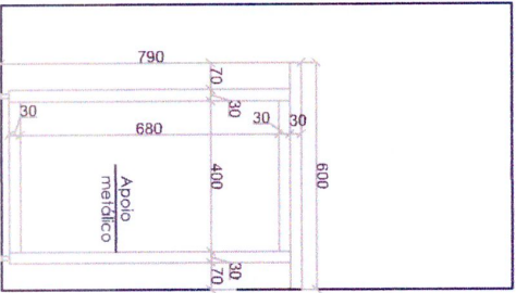
CORTE 1 - ESC. 1/50
