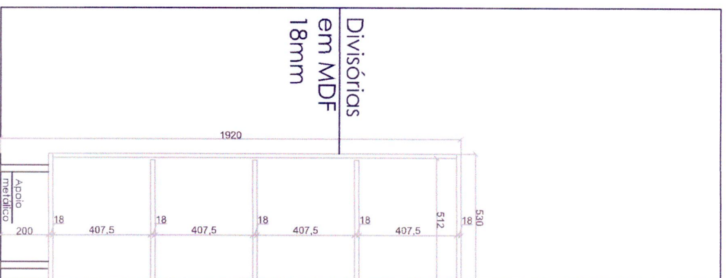
CORTE 5 - ESC. 1/50
