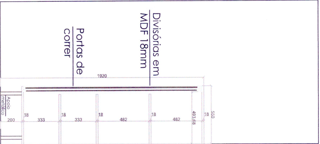
CORTE 6 - ESC. 1/50
