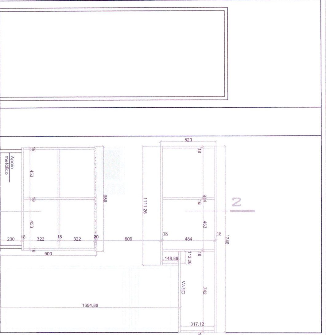
VISTA 2 ESC. 1/50
