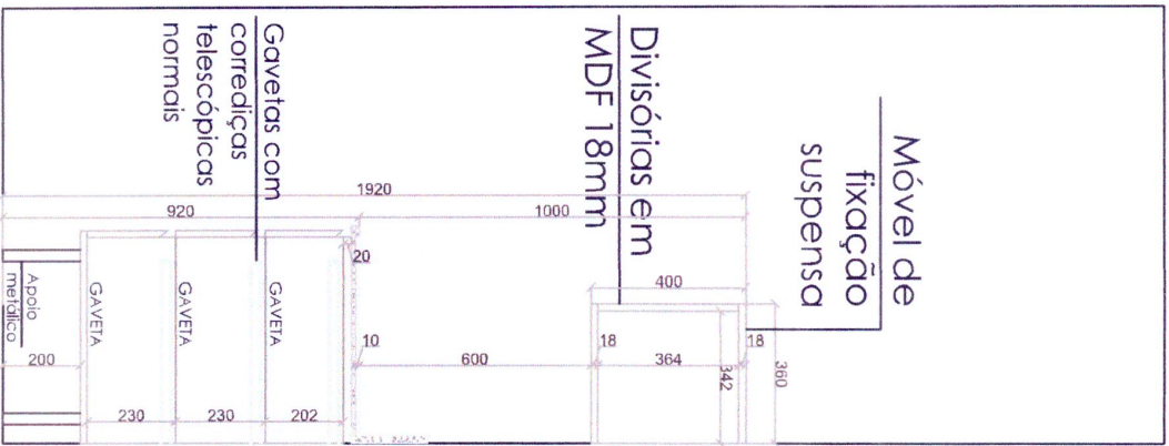
CORTE 7 - ESC. 1/50
