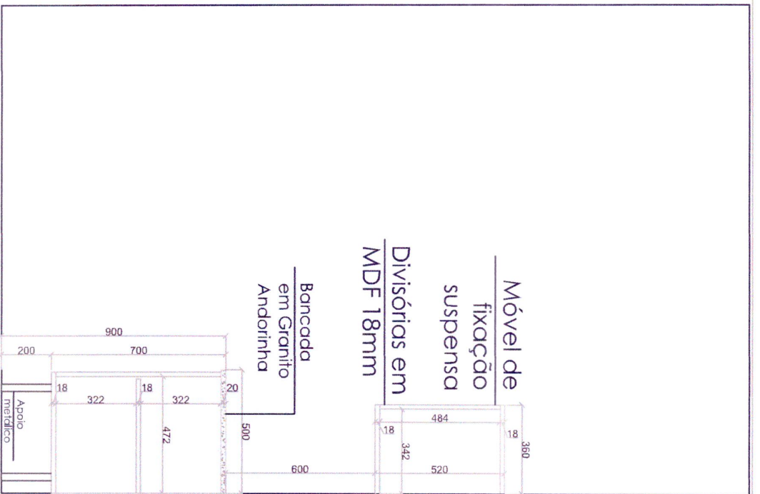
CORTE 2 - ESC. 1/50
