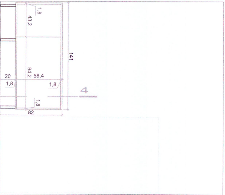
Vista interna - Móvel 02 Esc. 1/25
