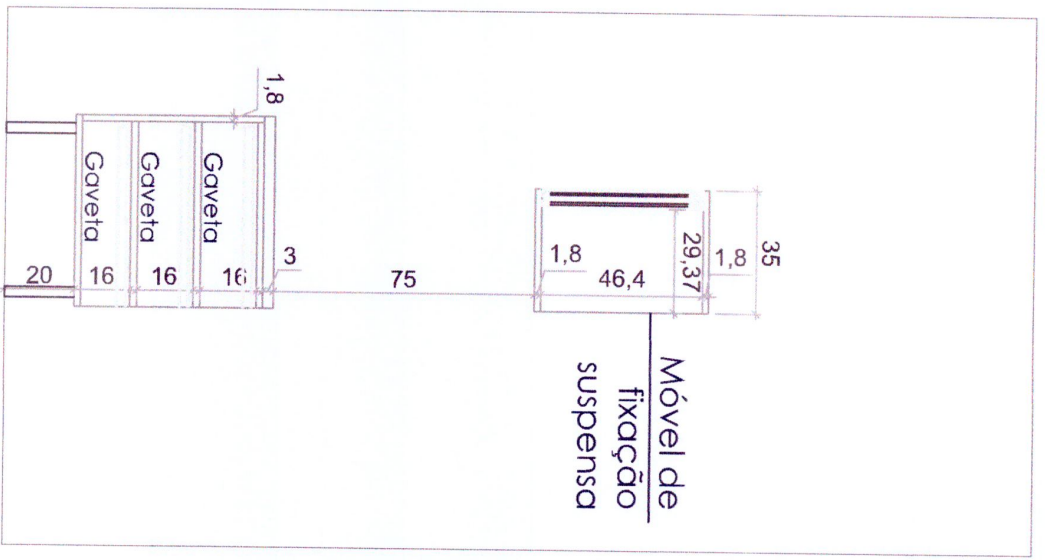
Corte 06 - Móvel 04 Esc. 1/20
