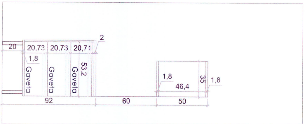
Corte 10 - Móvel 03 Esc. 1/20
