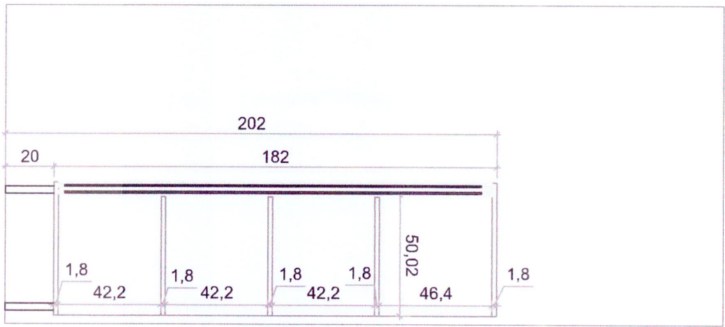
Corte 07 - Móvel 04 Esc. 1/20
