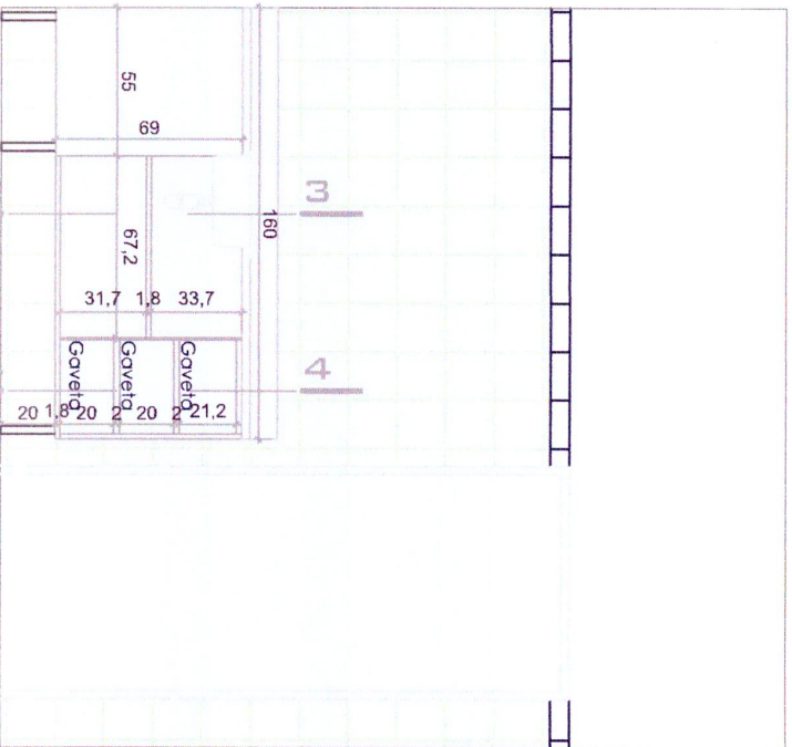
Vista 2 interna - Móvel 01 Esc. 1/25
