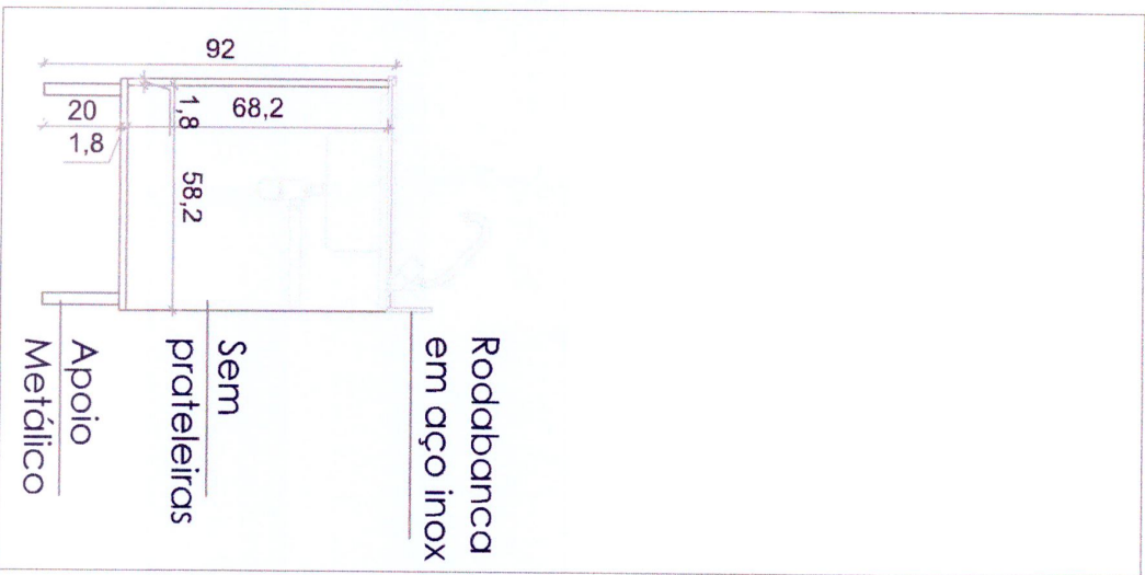
Corte 08 - Móvel 03 Esc. 1/20
