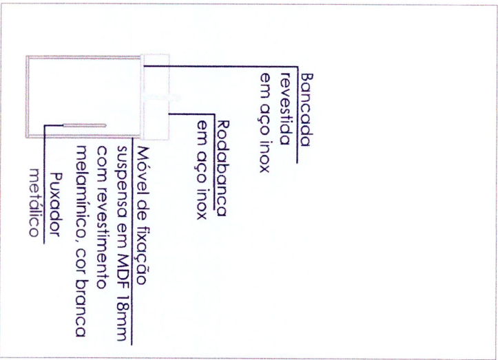
Vista 01 - Móvel 01 Esc. 1/25
