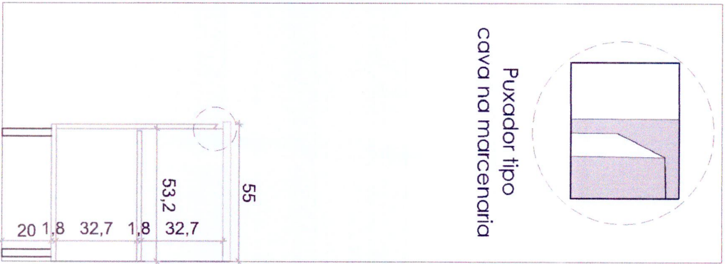
Corte 01 - Móvel 01 Esc. 1/20
