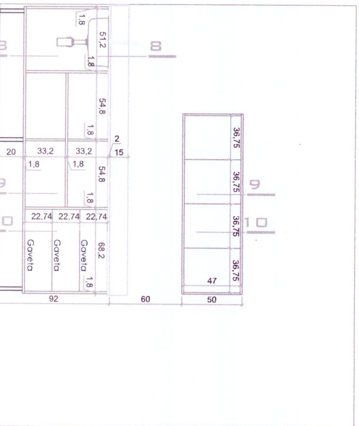
Vista interna - Móvel 03 Esc. 1/25
