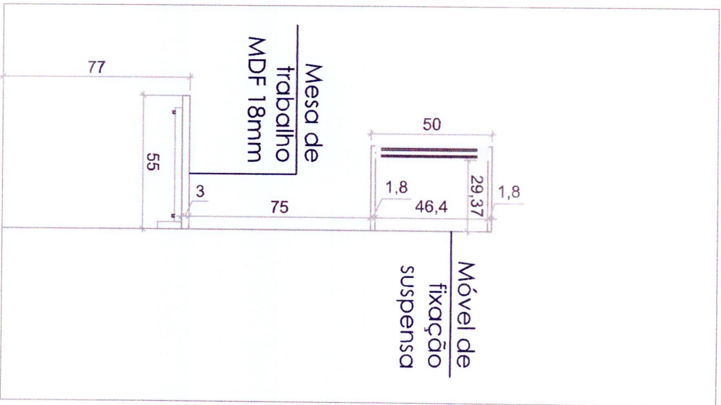
Corte 05 - Móvel 04 Esc. 1/20
