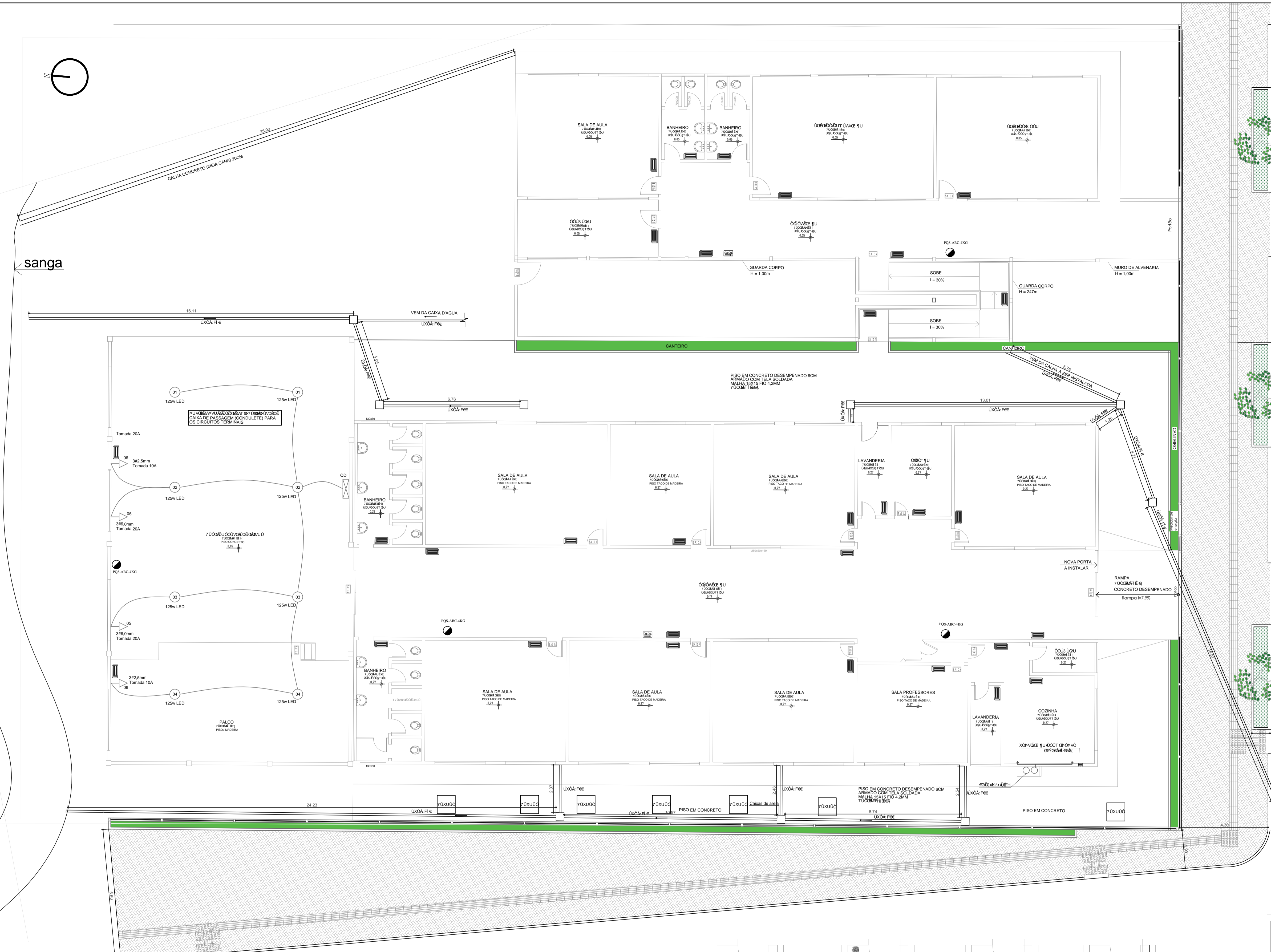
Planta Baixa - Passeio e Locação das grades Esc. 1/75
