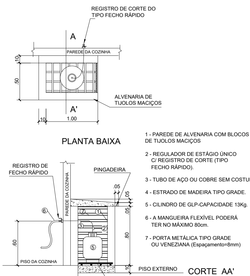
ABRIGO PARA BOTTIÃO DE GLP-13Kg
