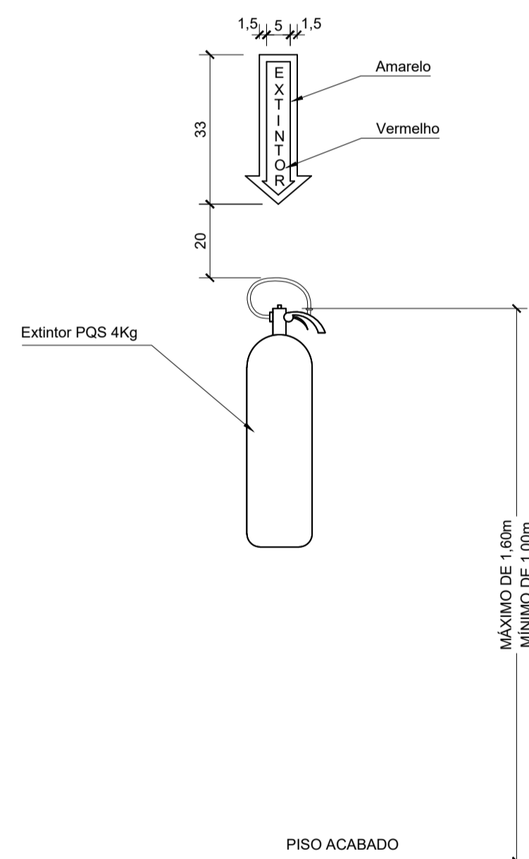
DETALHE DA INSTALAÇÃO Escala: 1/50
