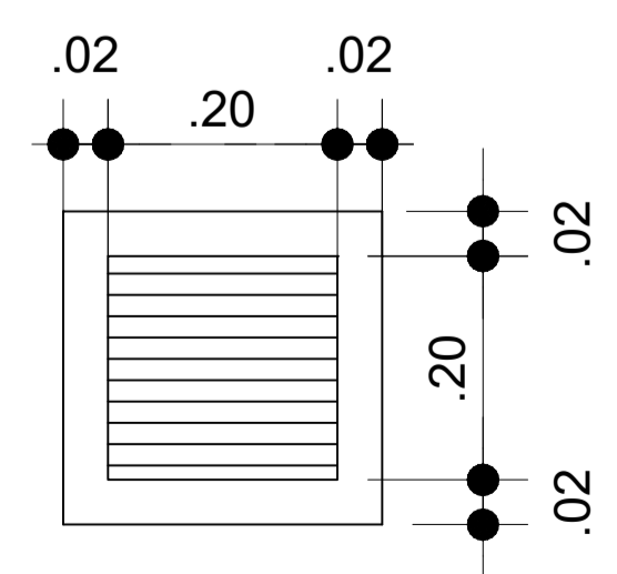
DETALHE DA VENEZIANA DA VENTILAÇÃO PERMANENTE ESCALA: 1/30
