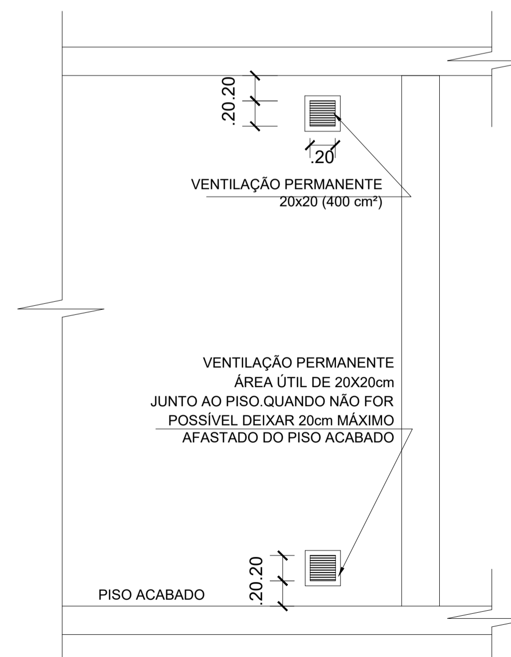
VENTILAÇÃO PERMANENTE (Adequação de ambiente) ESCALA: 1/30
