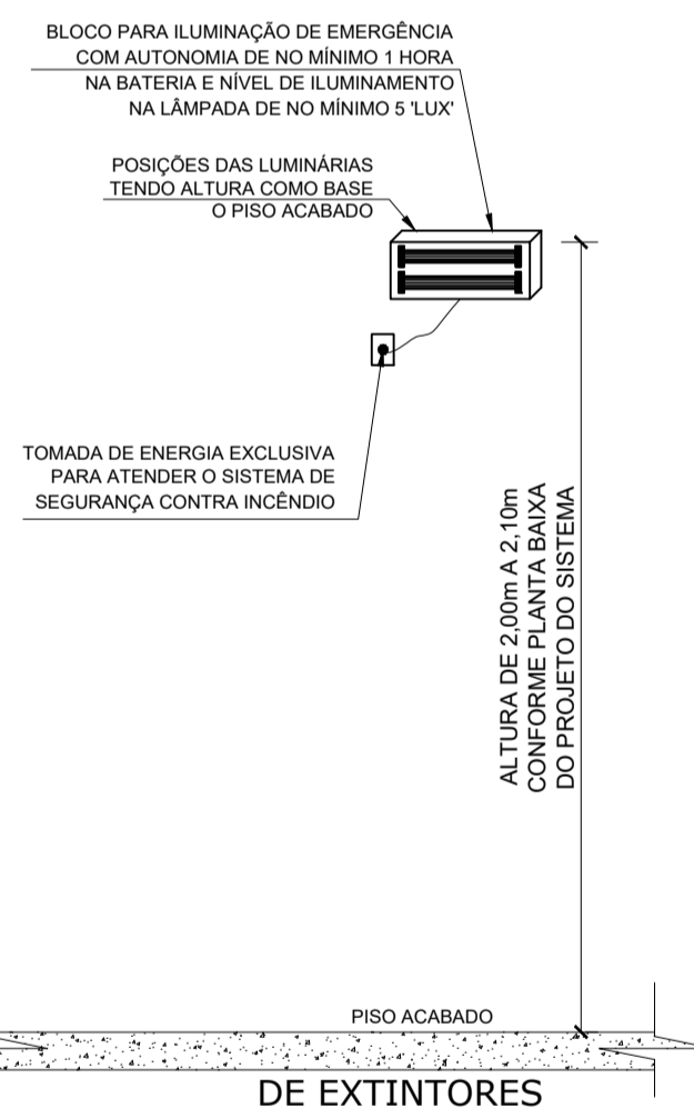
DETALHE DE INSTALAÇÃO DA ILUMINAÇÃO DE EMERGÊNCIA COM DUAS LÂMP FLUOR DE 8 W OU 30 LEDS Escala: 1/50
