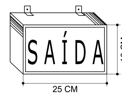
LUMINÁRIA TIPO BLOCO AUTÔNOMO DE ORIENTAÇÃO DE ABANDONO DE LOCAL (UMA FACE SEM SETA). ESCALA: 1/30
