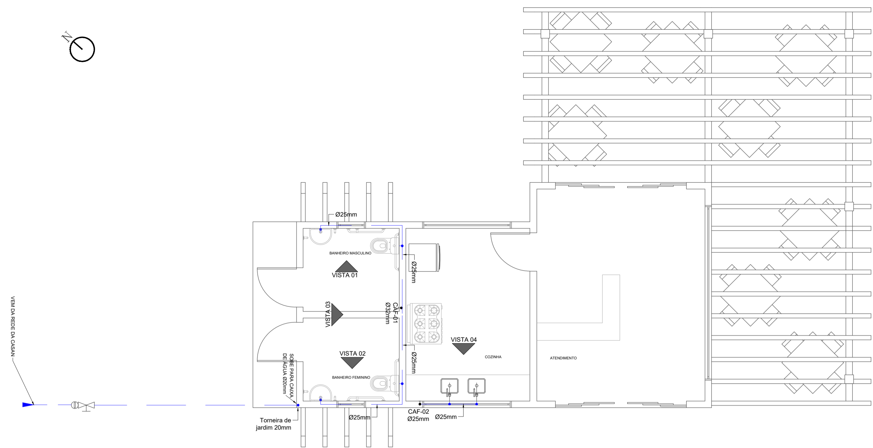
PLANTA BAIXA HIDRÁULICA ESCALA: 1/50
