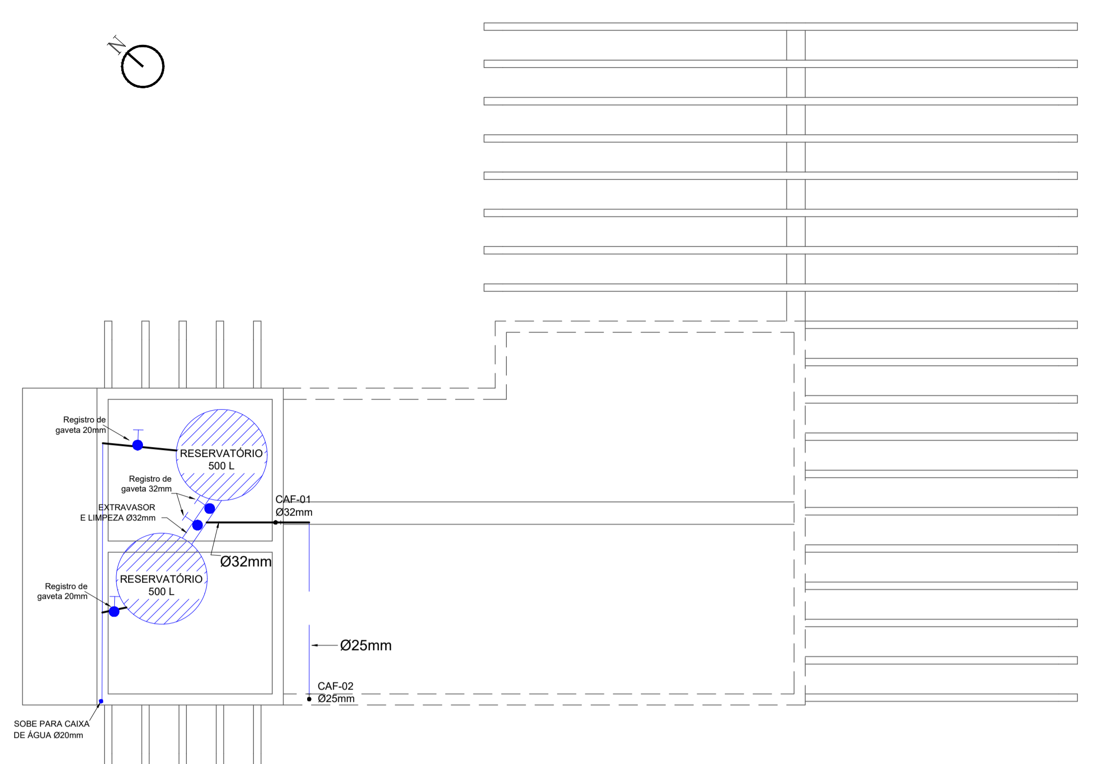
PLANTA COBERTURA HIDRÁULICA ESCALA: 1/50
