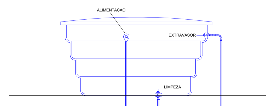
INSTALAÇÃO DE CAIXA D'ÁGUA CORTE TRANSVERSAL S/ESCALA
