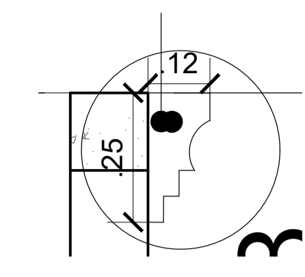
DETALHE PINGADEIRA ESCALA 1/10
