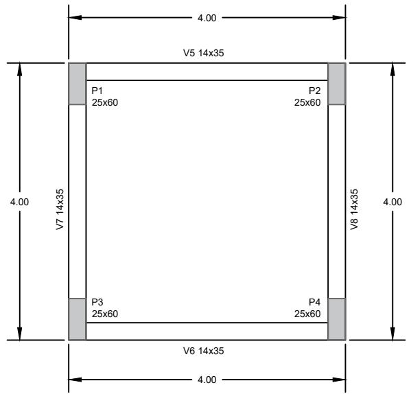
PLANTA DE FORMA NÍVEL 4,50 - VIGAS INTERMEDIÁRIAS ESC. 1/75
