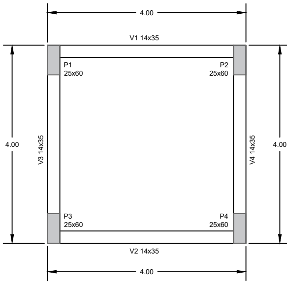
PLANTA DE FORMA NÍVEL 0,00 - VIGAS BALDRAME ESC. 1/75
