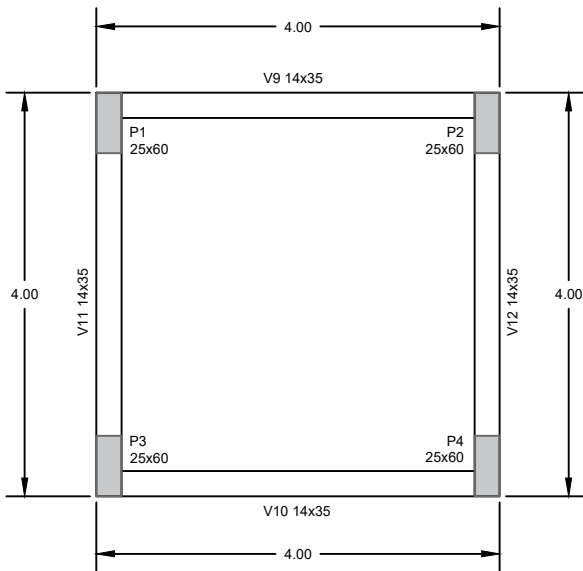
PLANTA DE FORMA NÍVEL 9,00 - VIGAS INTERMEDIÁRIAS ESC. 1/75
