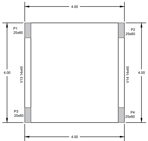
PLANTA DE FORMA NÍVEL 12,75 - VIGAS NÍVEL DA LAJE ESC. 1/75
