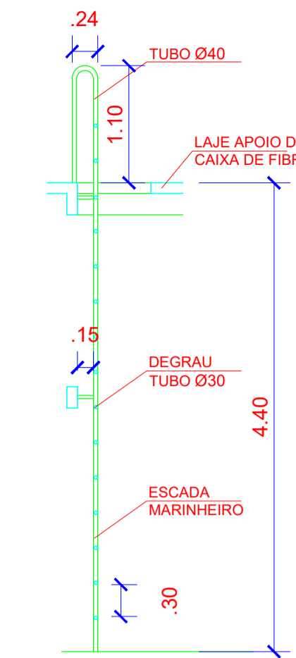
VISTA LATERAL ESCADA MARINHEIRO ESCALA 1/50
