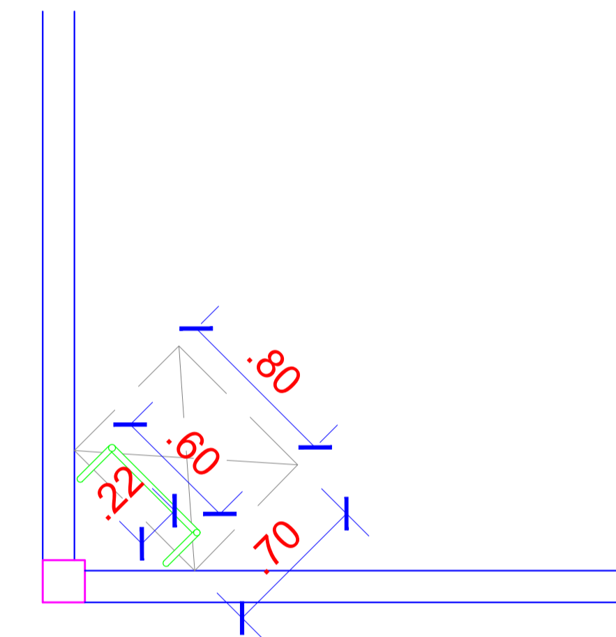
PLANTA SUPERIOR ESCADA MARINHEIRO ESCALA 1/25
