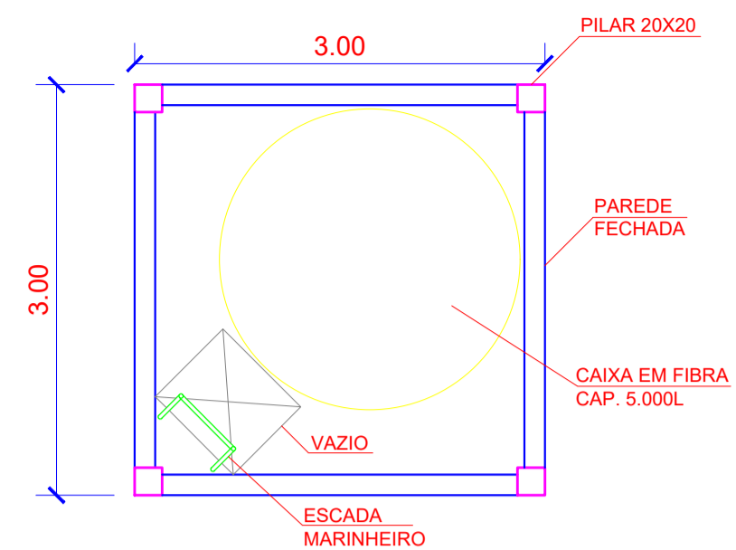
PLANTA SUPERIOR CASTELO D'ÁGUA CONCRETO ESCALA 1/50
