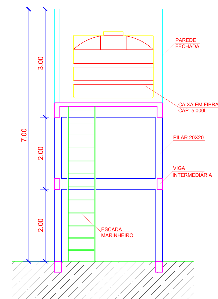
CORTE AA CASTELO D'ÁGUA CONCRETO ESCALA 1/50
