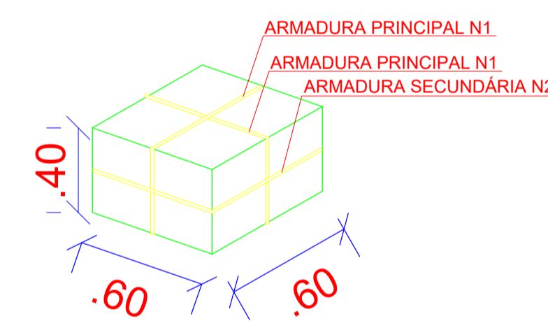
DETALHE ESTRUTURAL CAIXA D'ÁGUA ESCALA 1/50
