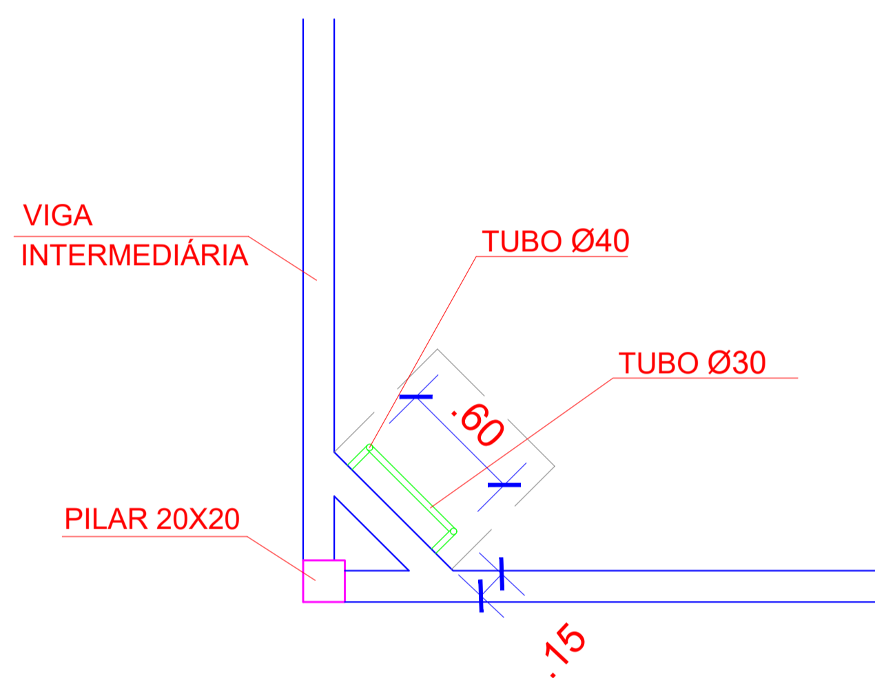
PLANTA INFERIOR ESCADA MARINHEIRO ESCALA 1/25
