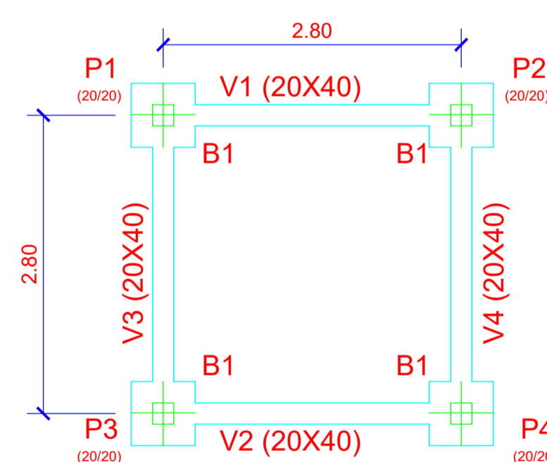
PLANTA INFERIOR ESCADA MARINHEIRO ESCALA 1/25
