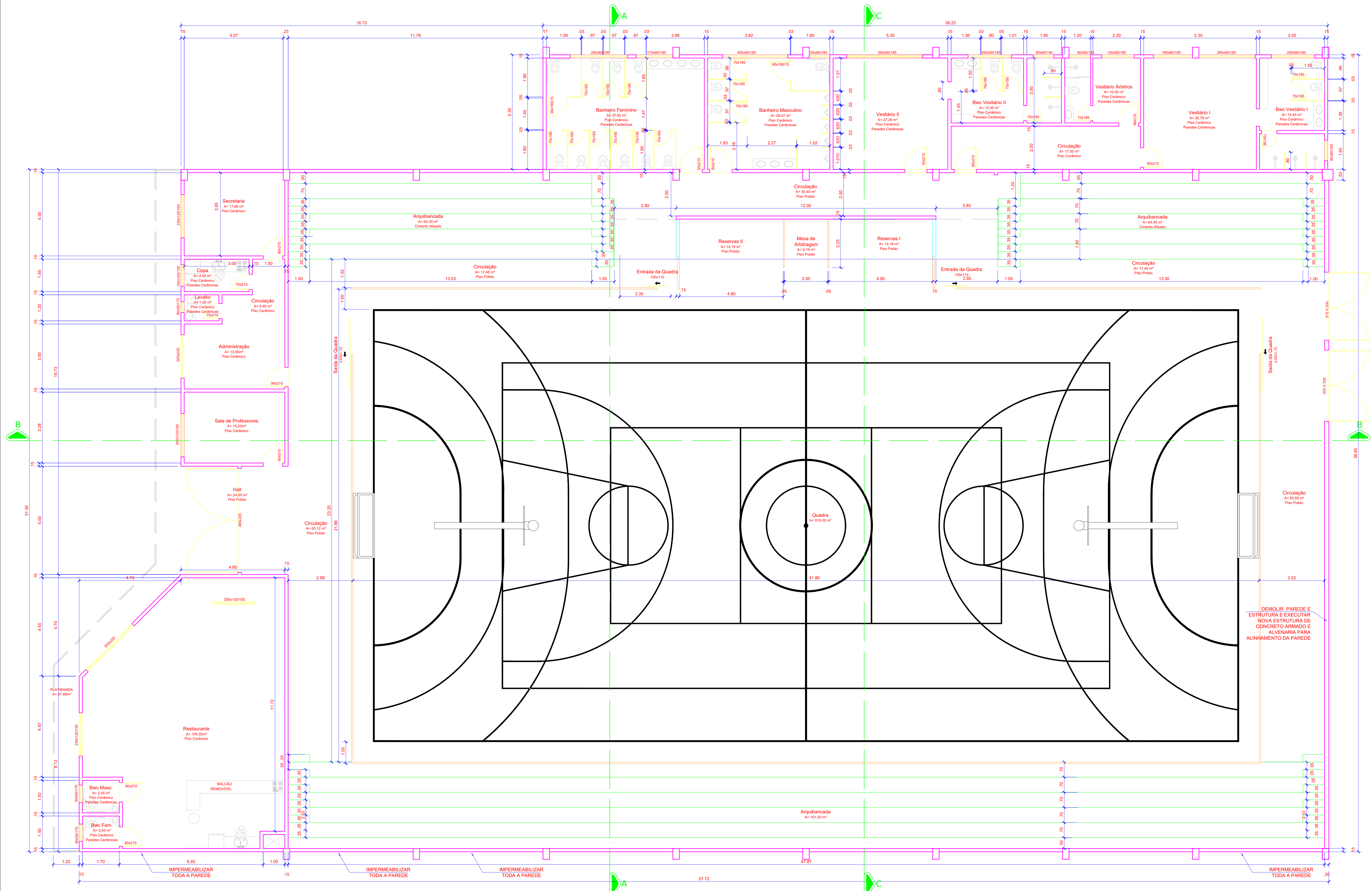
PLANTA BAIXA ESCALA: 1/75 ÁREA: 1.914,53m 2
