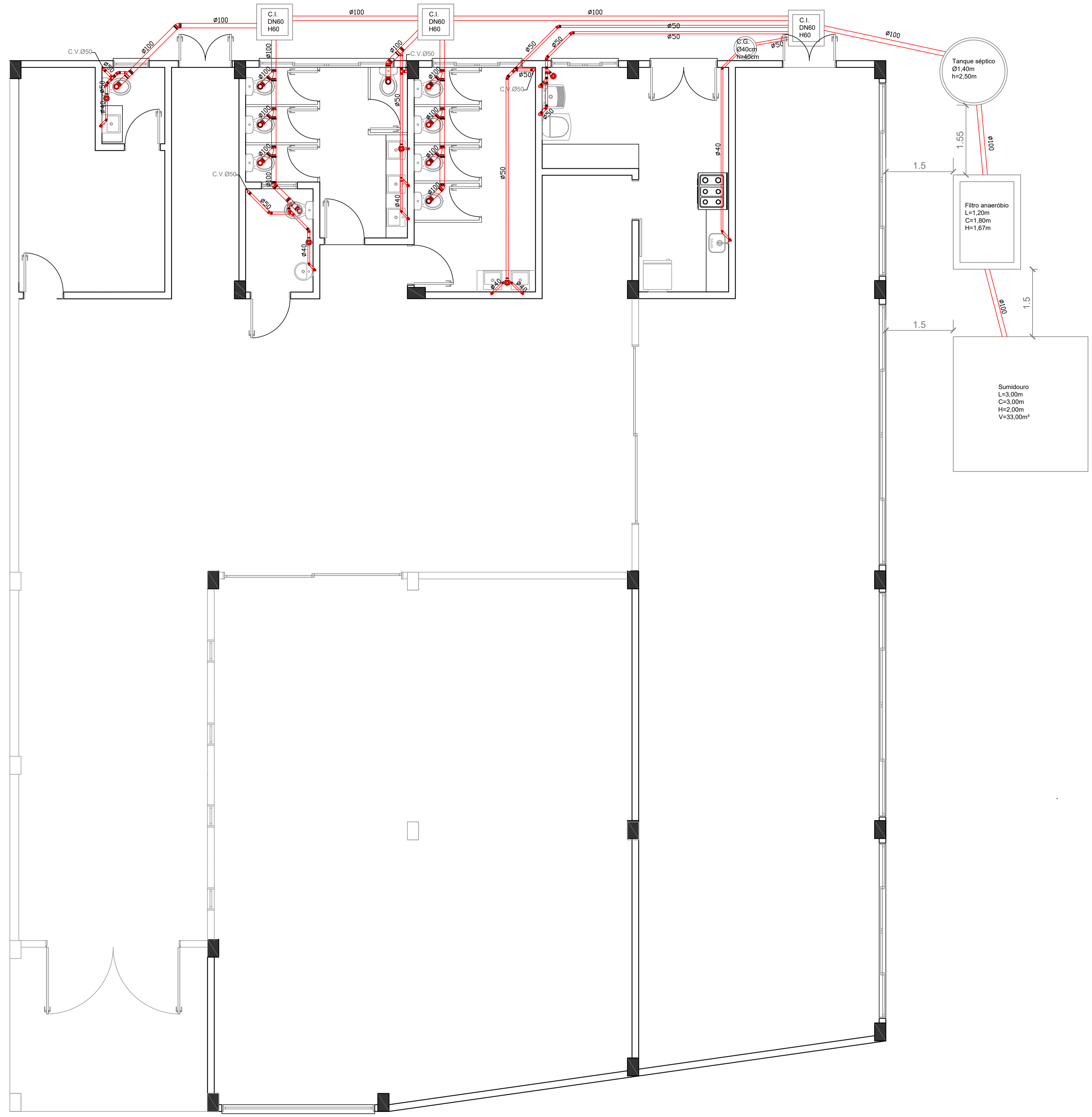
1 PLANTA BAIXA SISTEMA DE ESGOTO ESCALA 1/50
