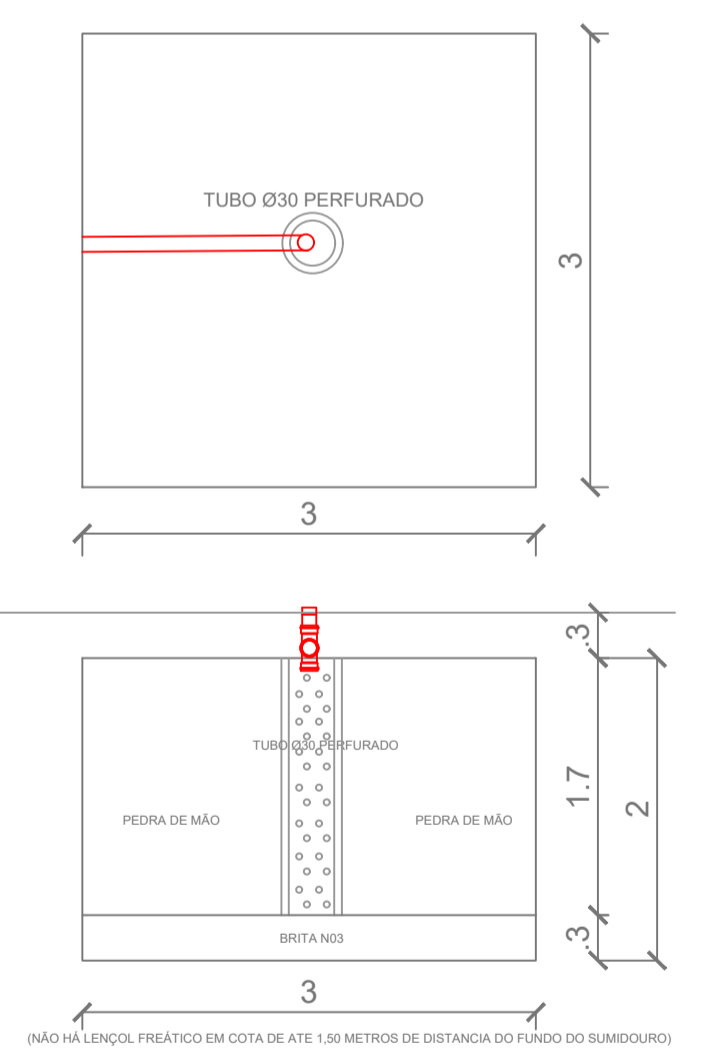
DETALHE DO SUMIDOURO ESCALA: 1/25
