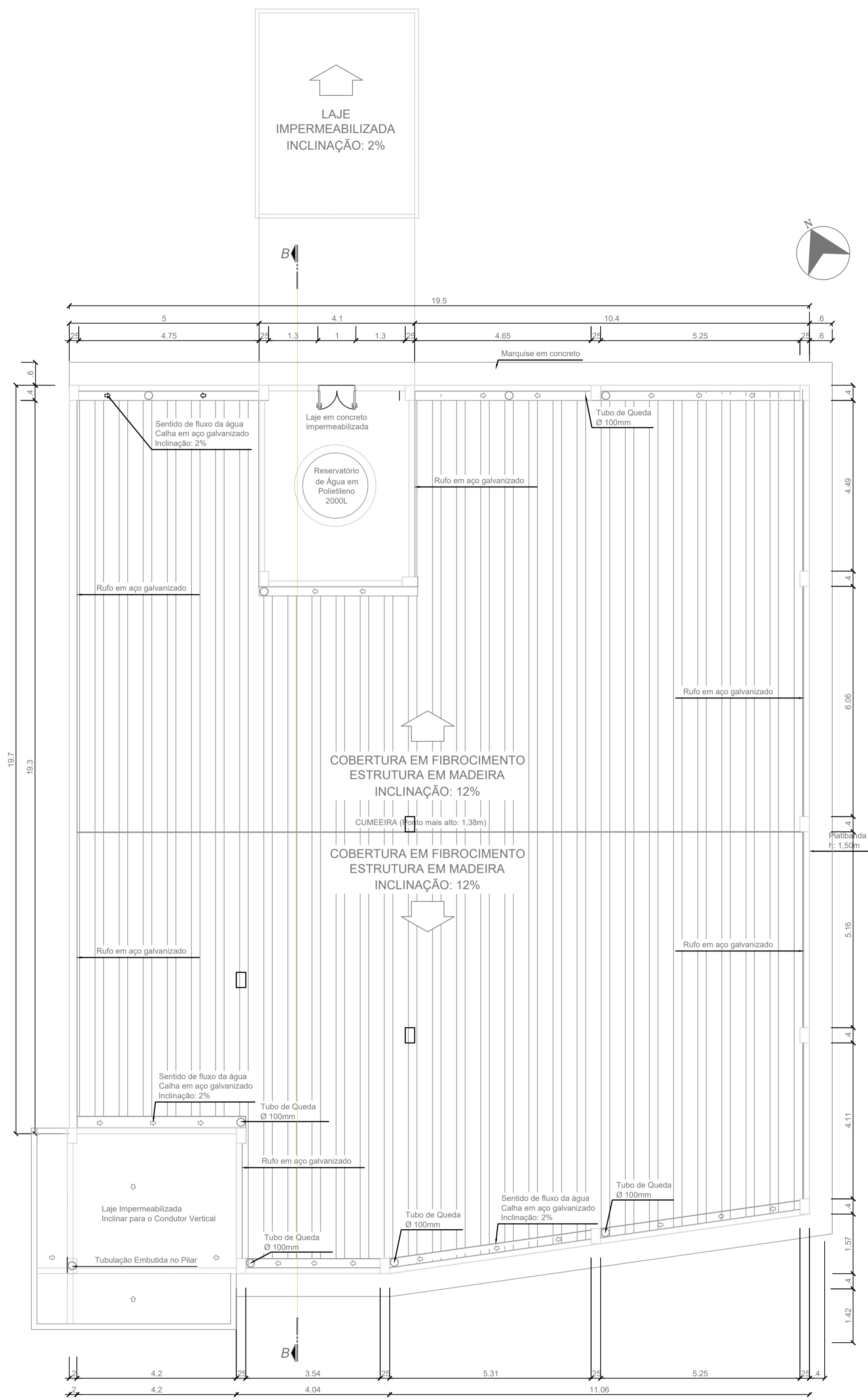
5 PLANTA DE COBERTURA ESCALA 1/75
